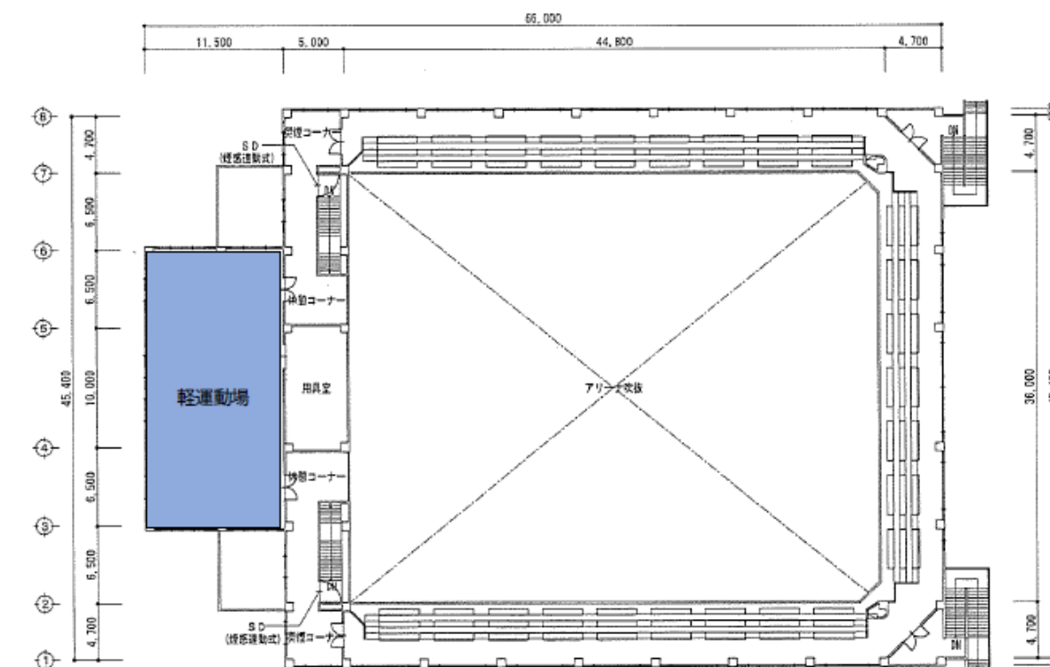
白沢体育館2階平面図
